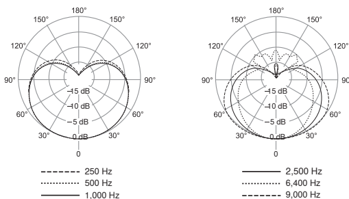
Patrón polar
